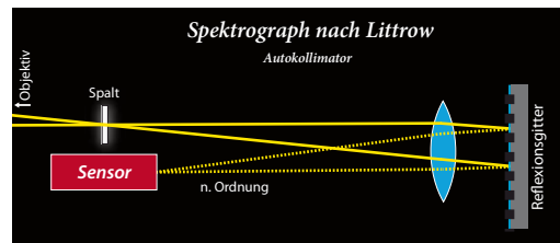
Abbildung 6.4 Spaltspektrograph mit Reflexionsgitter und Autokollimator (Bauweise nach Otto von Littrow). Durch Drehung des Gitters werden verschiedene Teile des Spektrums auf den Sensor gelenkt.
