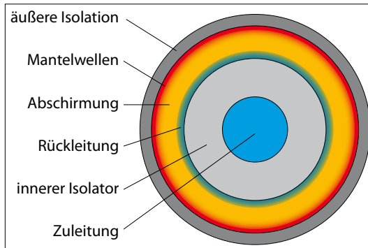
Aufbau eines Koaxkabels.
